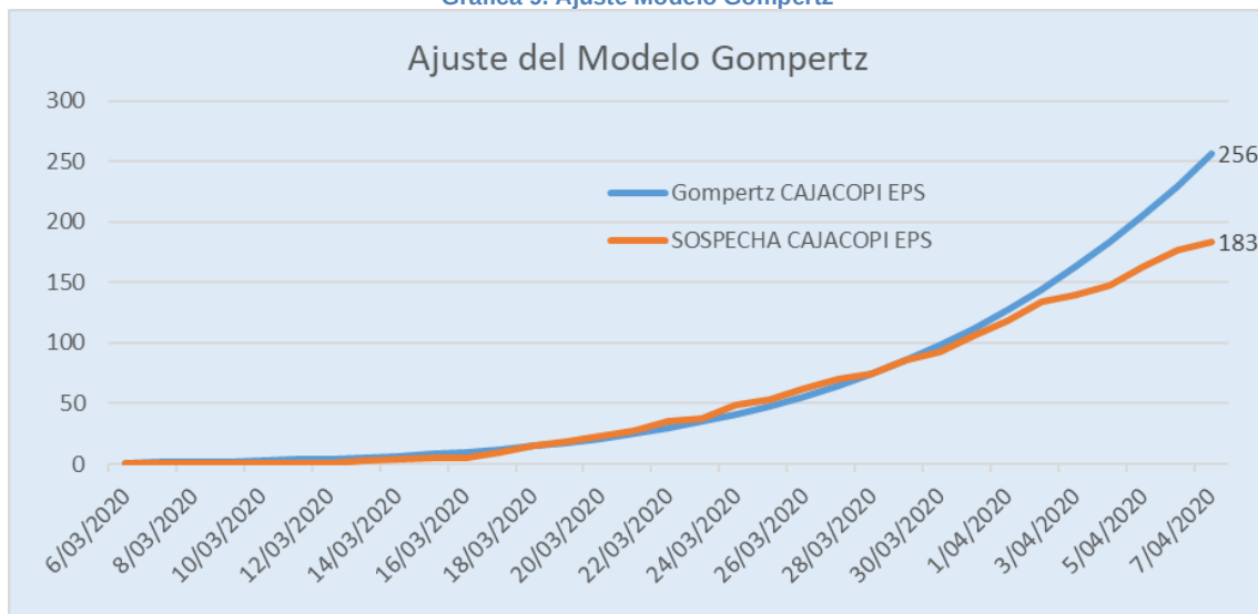
Gráfica 9. Ajuste Modelo Gompertz
