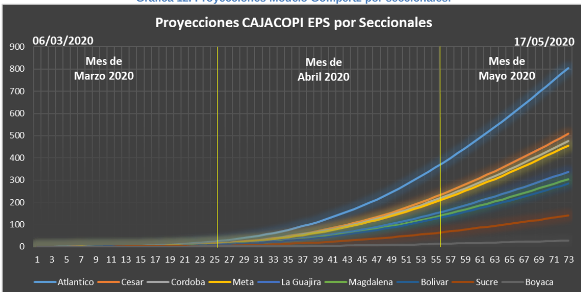
Gráfica 12. Proyecciones Modelo Gompertz por seccionales.
