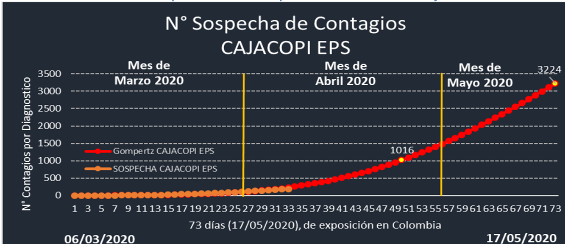
Gráfica 10. Comportamiento casos reportados reales Vs. Casos Proyectados
