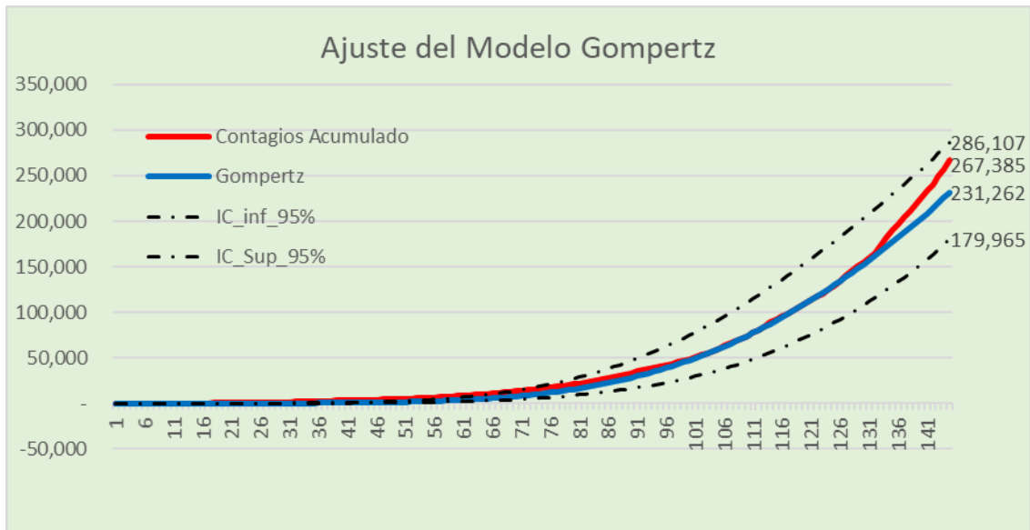
Gráfica 14. Ajuste del Modelo Gompertz
