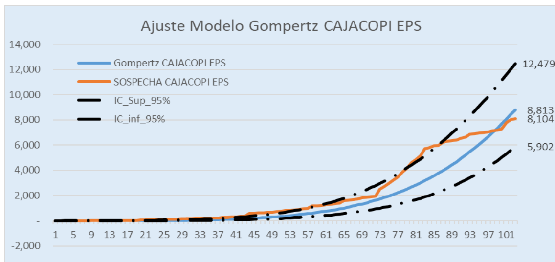
Gráfica 16. Modelo Ajustado para los últimos 15 días del mes de junio 2020.
