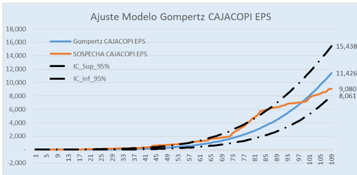
Gráfica 14. Ajuste Modelo Gompertz Cajacopi EPS
