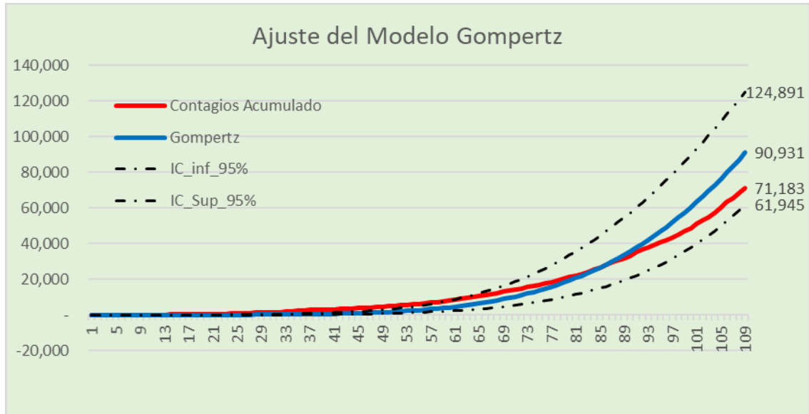
Gráfica 13. Ajuste Modelo Gompertz
