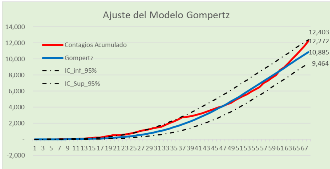
Gráfico 16. Ajuste del Modelo Gompertz
